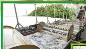
▲後成環保有限公司新購建的塑膠清洗系統，可以自動分辨PET及HDPE塑膠，大大增加回收效率。
